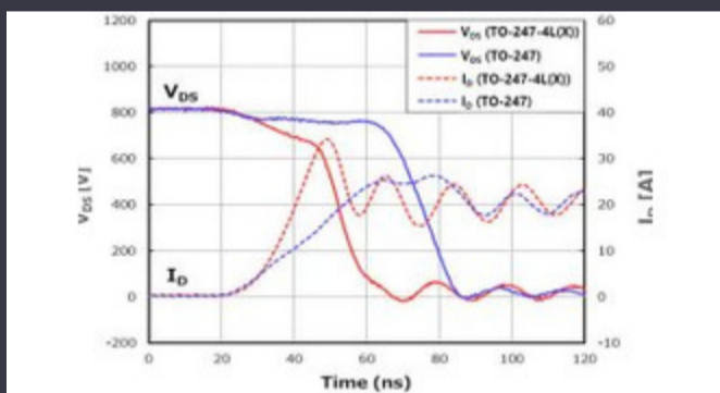
בן ארבע פינים כדי לחתוך הפסדים SIC MOSFET טושיבה מוסיף 2023/08/31
